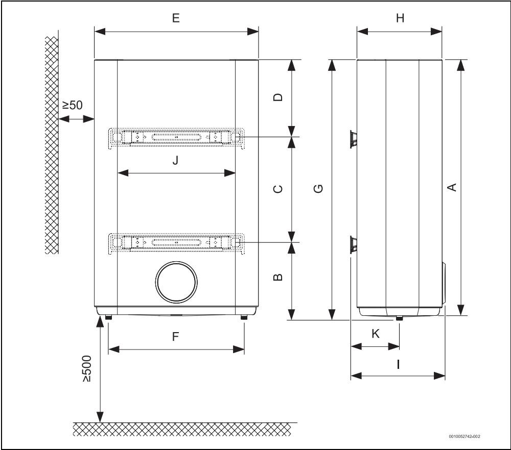
Фиг. 2 Размери в мм (стенен монтаж, вертикална инсталация)
